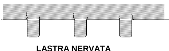
Figura 5.17: Nelle lastre nervate la fessurazione è dovuta all'assestamento differenziale dell'impasto.
